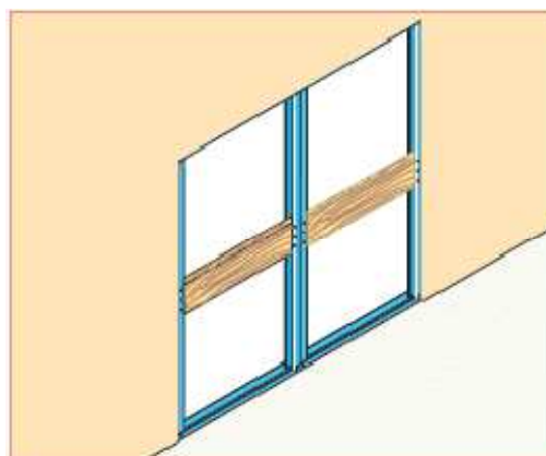
Passo 03 – Reforço de montantes
