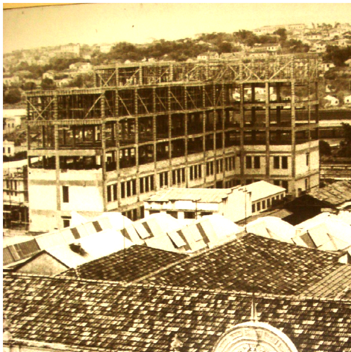
FIGURA 2 - Imagem da época da obra - Esquema estrutural Ed. Arthur Guimarães
